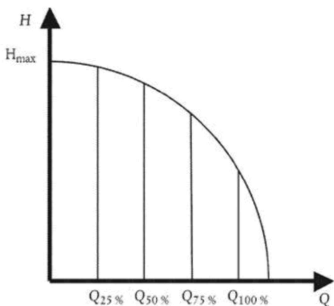
Рис. 3. Профиль нагрузки.
